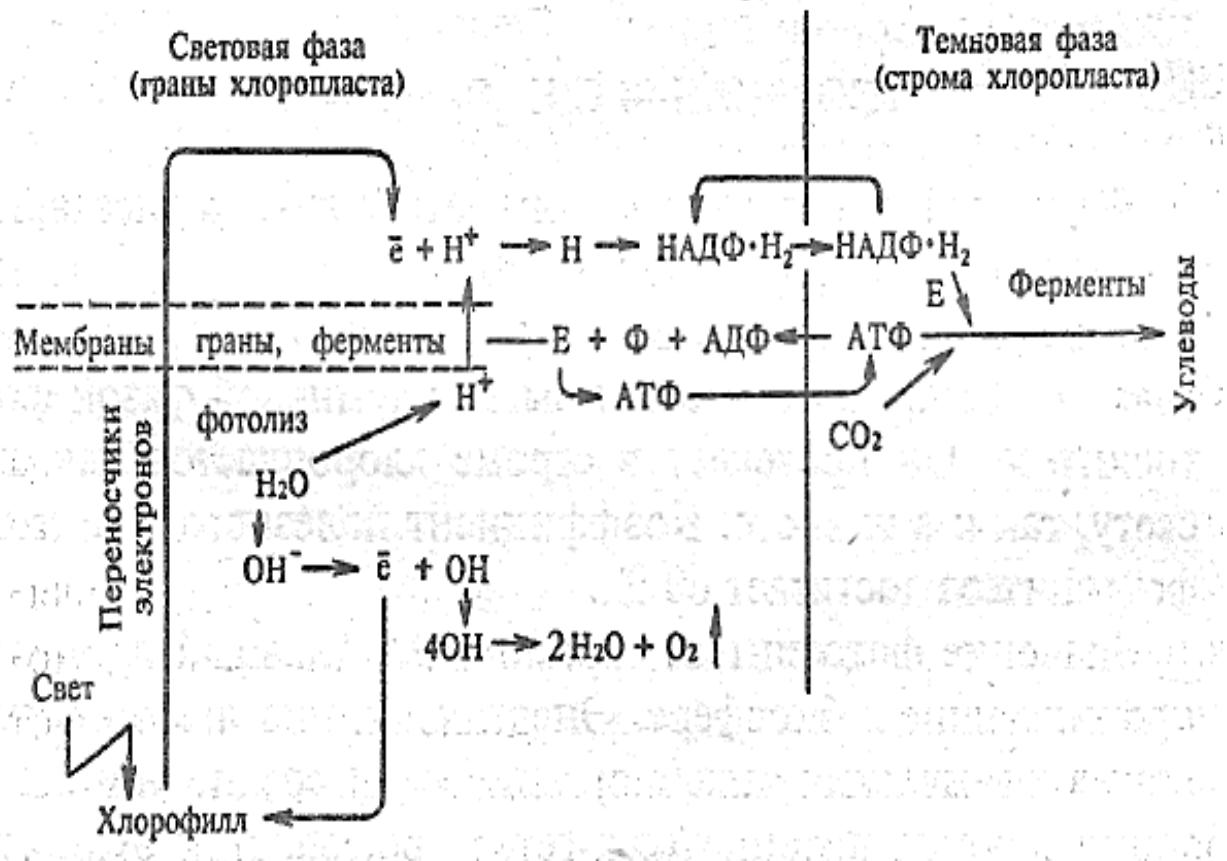
Рисунок 3 - Фазы фотосинтеза
