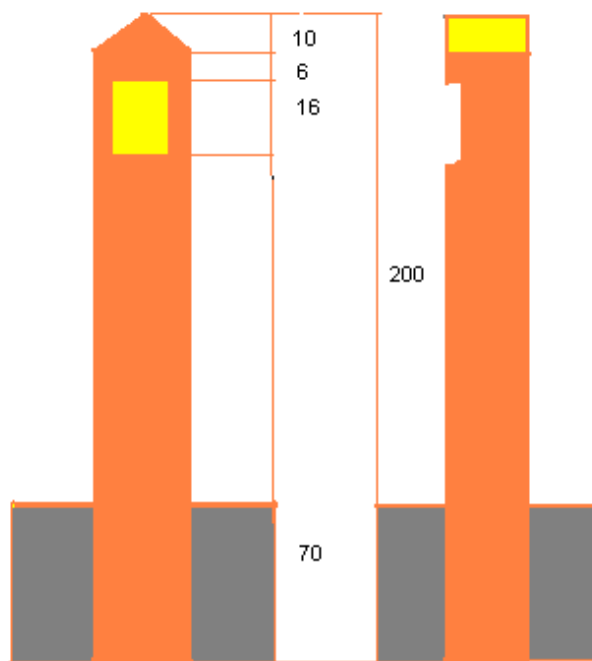
Рис. Лесосечный столб
