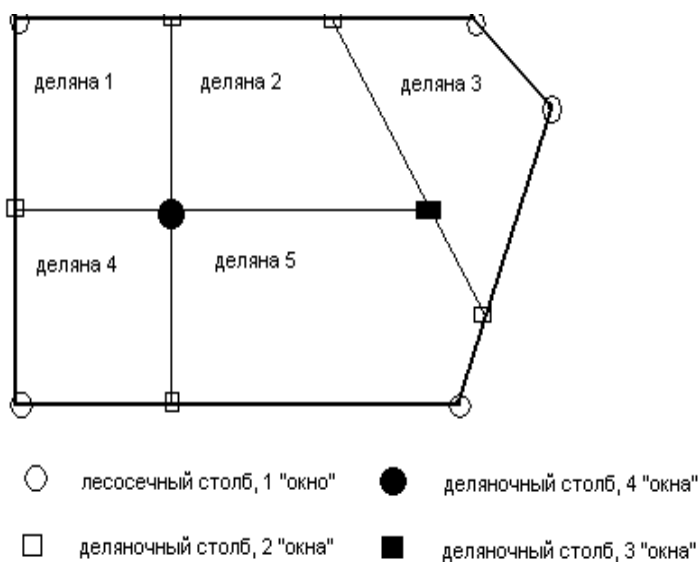
Рис. Места постановки лесосечных и деляночных столбов в лесосеке. Количество «окон» у них, в зависимости от места постановки.
