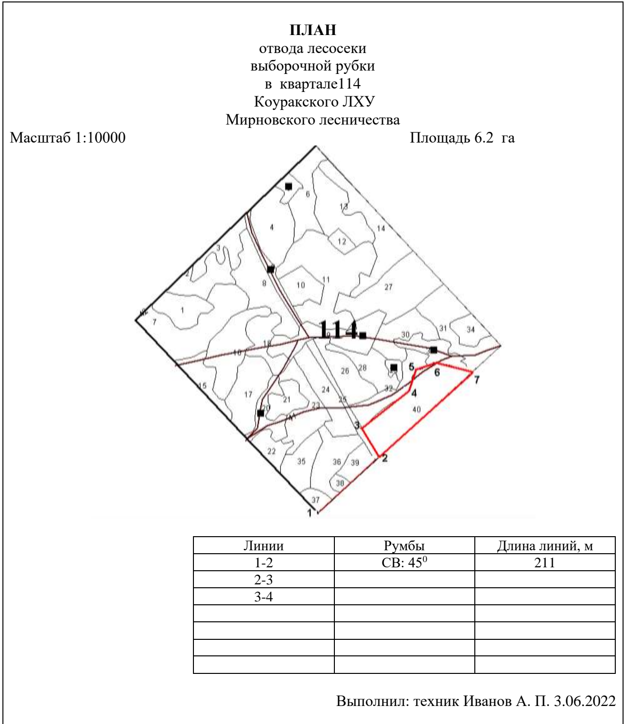
Рис. План отвода лесосеки
