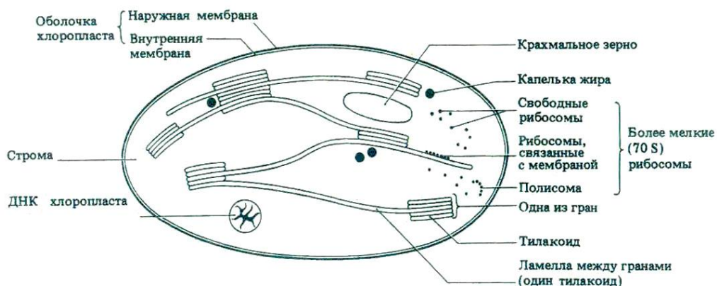
Рисунок 2 – Строение хлоропласта
