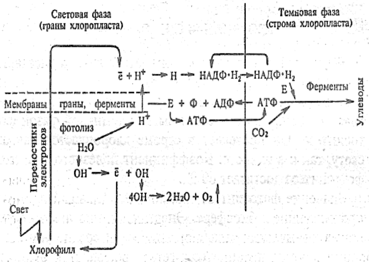
Рисунок 3 - Фазы фотосинтеза
