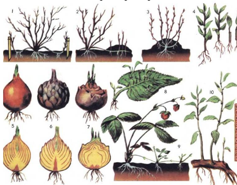
Рисунок 7. - Вегетативное размножение
