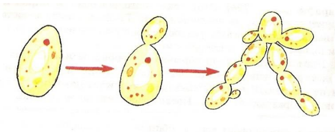
Рисунок 8. - Почкование
